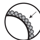
内弯最小半径 R 400 Internal curve R min. 400
