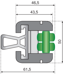
铝侧板 Aluminum Profile
