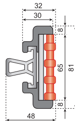
铝侧板 Aluminum Profile
