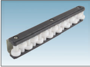
RG901 单排算盘护栏 RG901 SIMPLEX ROLLER GUIDE
