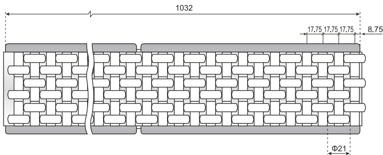
RG903 三排算盘护栏 RG903 TRIPLEX ROLLER GUIDE
