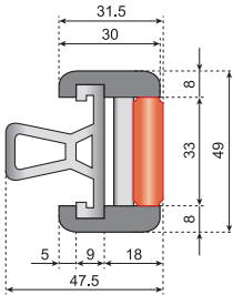
铝侧板 Aluminum Profile
