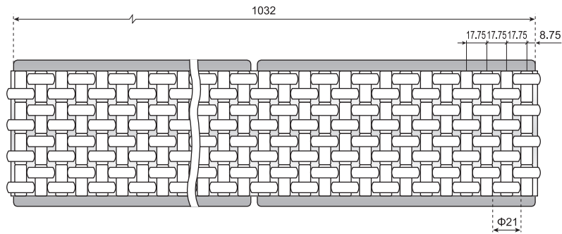
RG904 四排算盘护栏 RG904 QUADRUPLICATE ROLLER GUIDE
